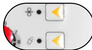
Función prueba alambre y gas en GMAW
